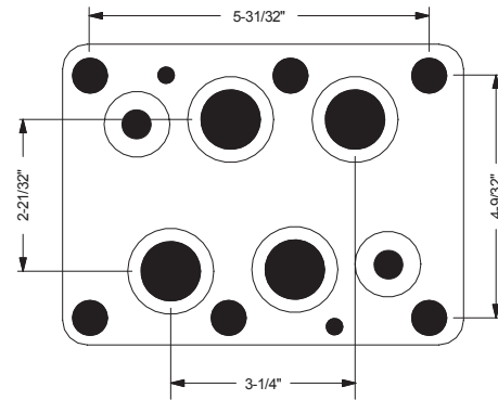
D08 Used on: DG5S4 06 DG3S4 06 DG5S8 DG5SH8 DG3S8 DG5V8 DG3V8 4WEH25 4WH25
