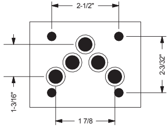
D05 Used on: DG4S4 01 DG4V4 01 DG4V5 4WE10
