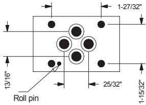
D03 Used on: DG4V 3 4WE6
