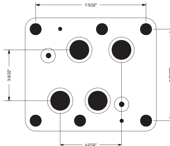
D10 Used on: DG17S4 10 DG5S4 10 DG3S4 10 4WEH32 4WH32
